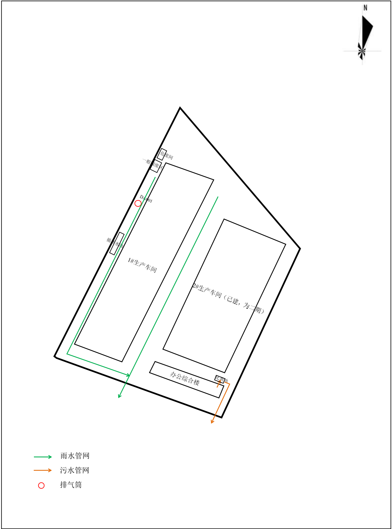
附图3 项目平面布置图及雨污管网图
